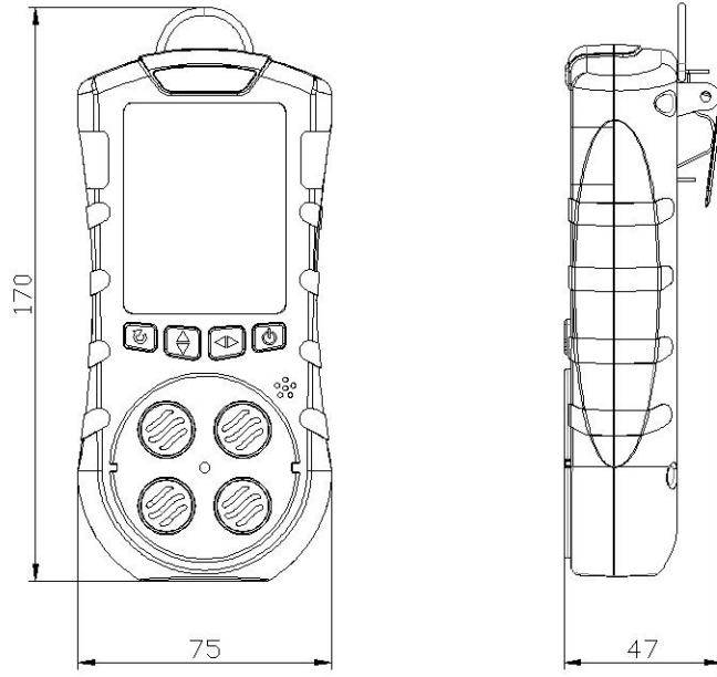
图 1 外型尺寸图
